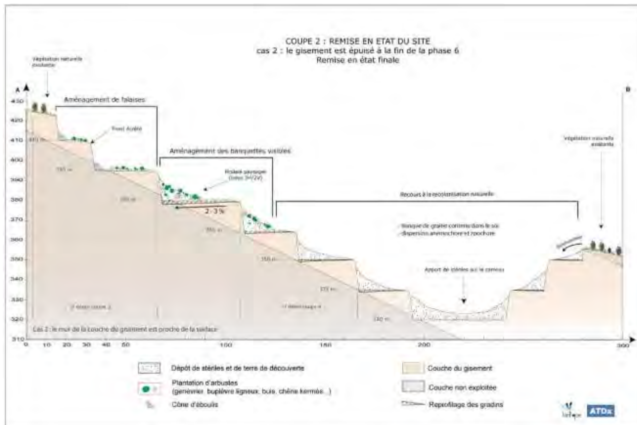
Figure 19 : Schéma de remise en état de carrière
